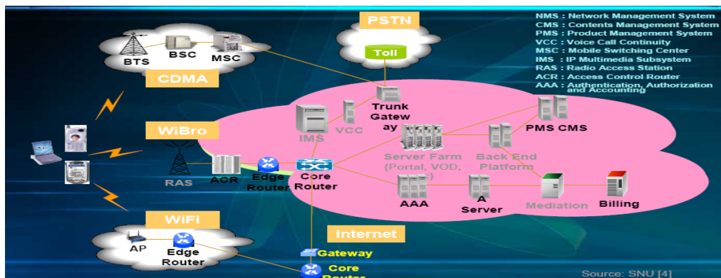
Gambar 2. Arsitektur Jaringan WIBRO (google.co.id)
