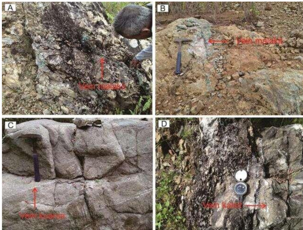
Gambar 6. Singkapan kekar tarik dilapangan pada Satuan marmer Tuhur terisi mineral malakit, azurit, kalsit dan kuarsa.
