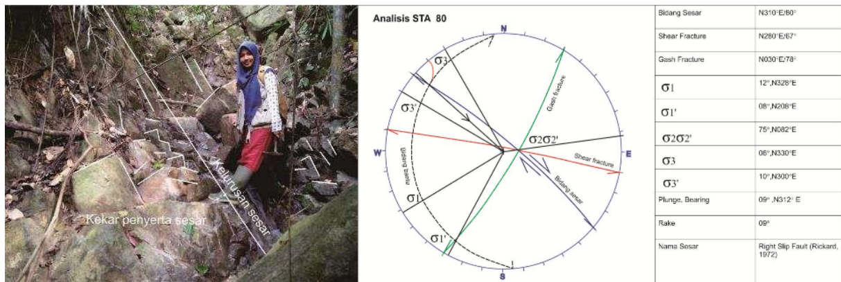
Gambar 9. Zona kelurusan Sesar dan kekar penyerta Sesar Bukit Bua yang memotong Satuan granodiorit Sult Air (Azimut foto: N 340°E) dan analisis stereografis Sesar Bukit Bua Sesar mendatar kiri berarah barat laut-tenggara (NW-SE)
